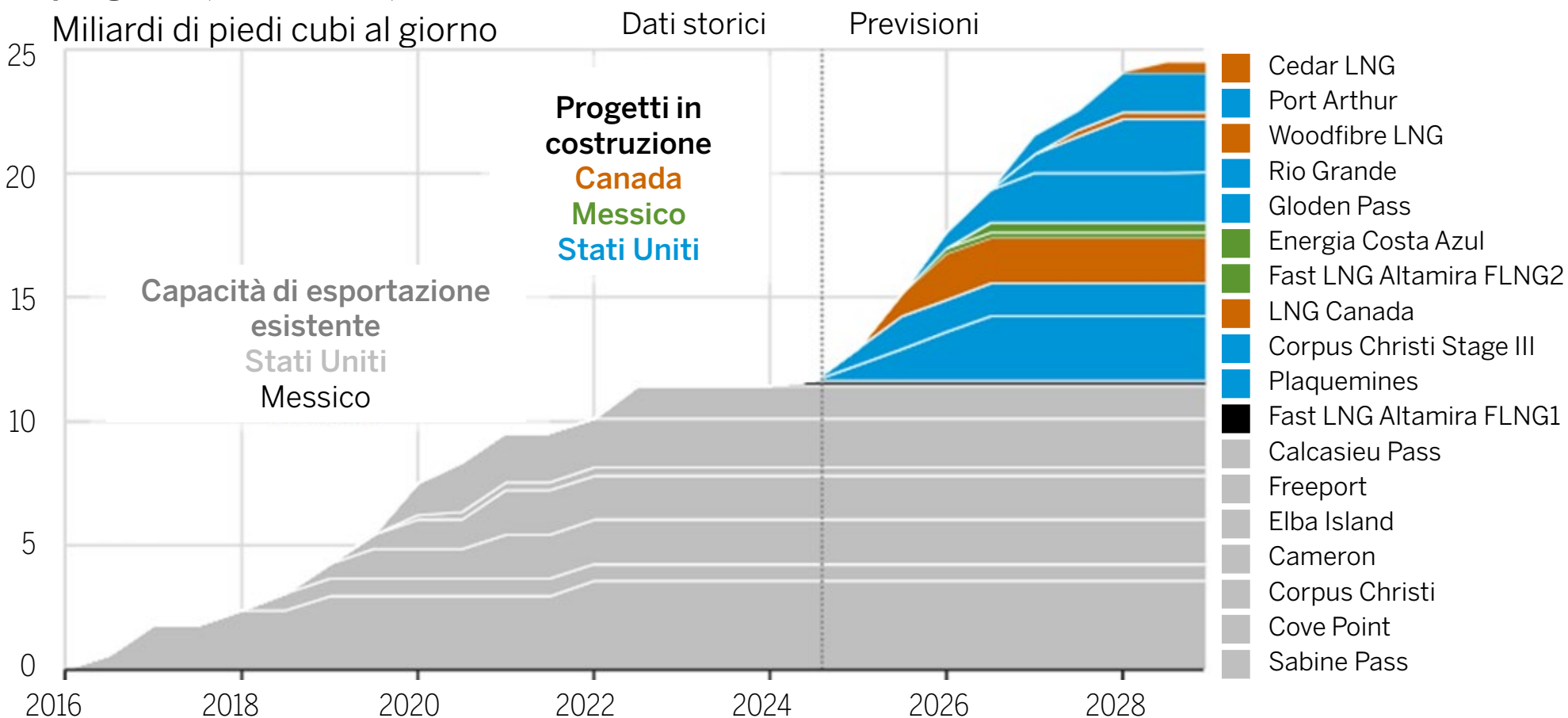
Capacità di esportazione di gas naturale liquefatto del Nord America per progetto (2016-2028)
